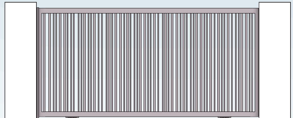
ARI 105 Portail Coulissant
